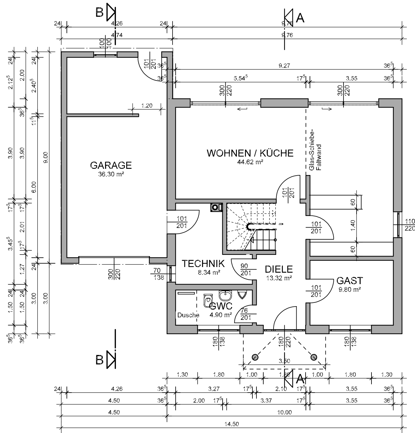
Grundriss EG
