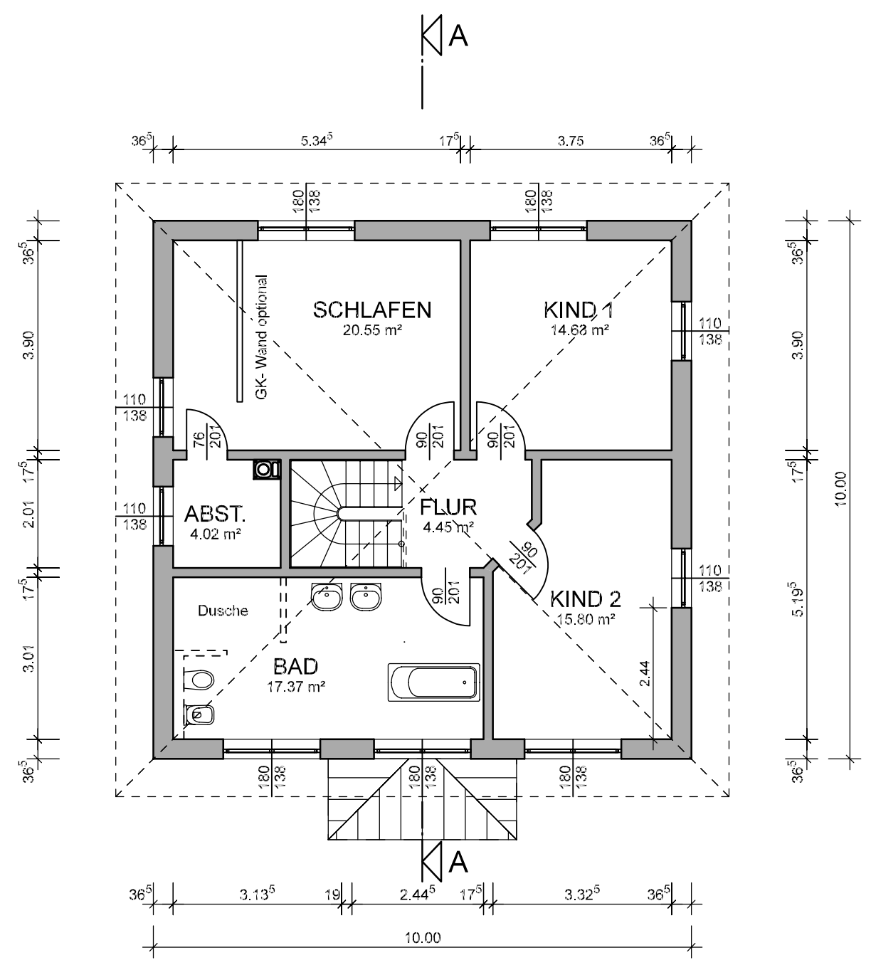
Grundriss OG
